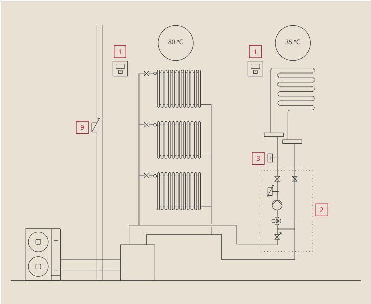
Remplacement de chaudière Chauffage 2 circuits
