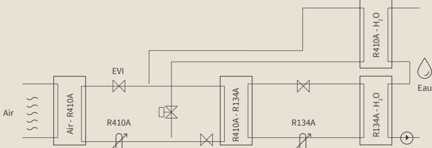
Fig. 1 : Schéma du cycle Smart Cascade
