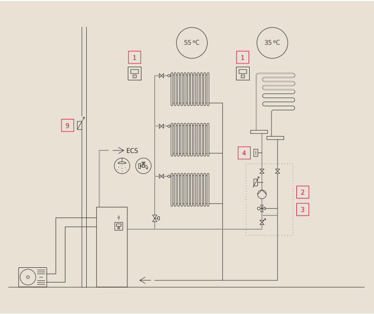
Chauffage 2 zones avec circuits radiateurs et plancher chauffant + ECS
