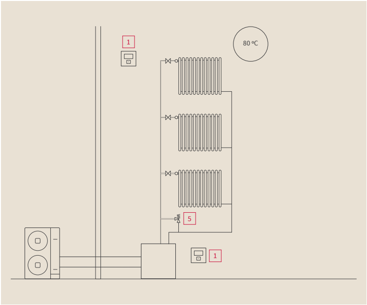
Remplacement de chaudière Chauffage 1 circuit
