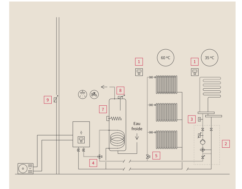
2 zones avec circuits radiateurs et plancher chauffant avec ou sans ECS
