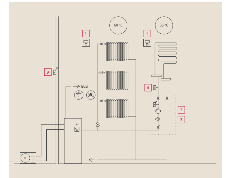
Chauffage 2 zones avec circuits radiateurs et plancher chauffant + ECS
