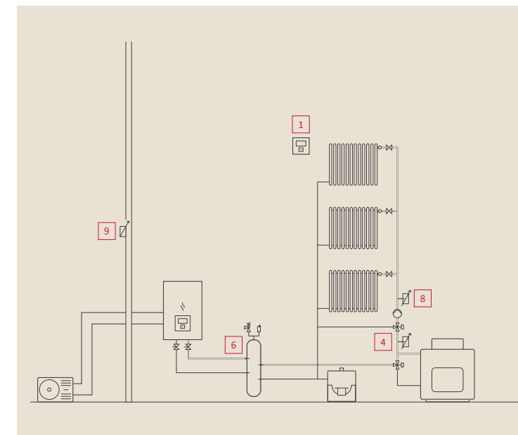
Relève chaudière 1 circuit radiateurs
