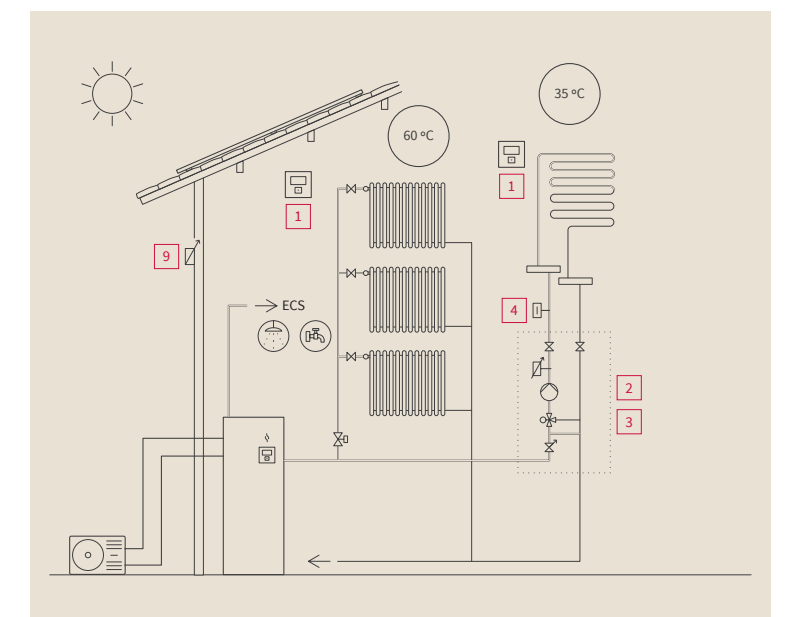
Chauffage 1 circuit radiateurs et plancher chauffant + ECS
