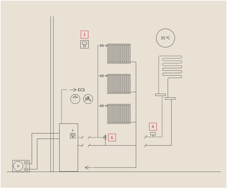
Chauffage 1 circuit radiateurs ou plancher chauffant + ECS
