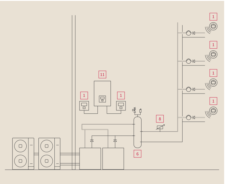
Remplacement de chaudière Cascade : application chauffage individuel centralisé
