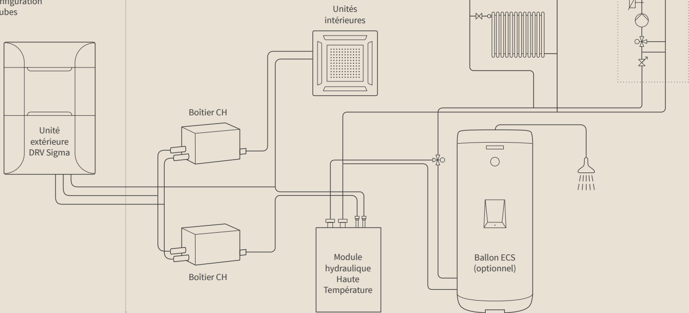
Exemple de configuration possible en 3 tubes
