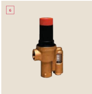
Soupape de décharge différentielle Cet accessoire garantit un débit constant au travers du condenseur de la PAC. ATW-DPOV-01
