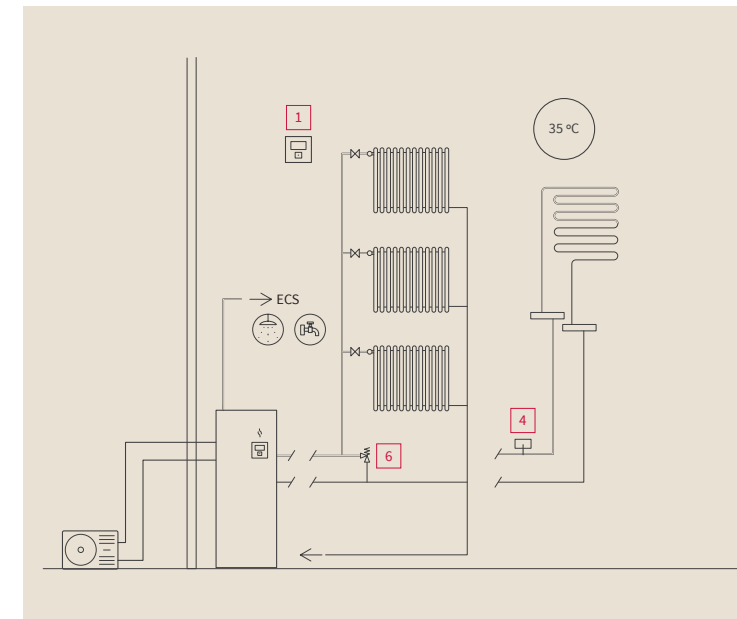
Chauffage 1 circuit radiateurs ou plancher chauffant + ECS
