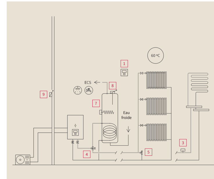
1 zone radiateurs ou plancher chauffant avec ou sans ECS
