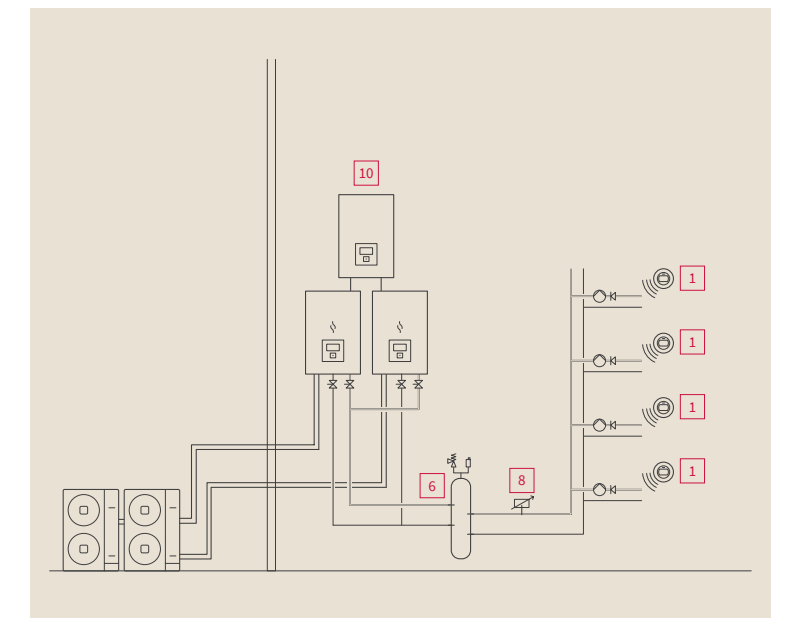
Cascade : application chauffage individuel centralisé
